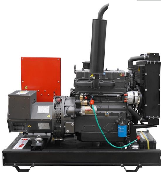
Kolektor wydechowy ze względu na budowę oraz umiejscowienie, posiada szeroki zakres zastosowania różnych układów wydechowych oraz systemów odprowadzenia spalin.
